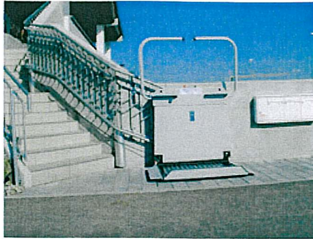
▶ T80 Outdoor system with hot-dip galvanized guide rails T80 installation extérieure avec rail galvanisé à chaud
